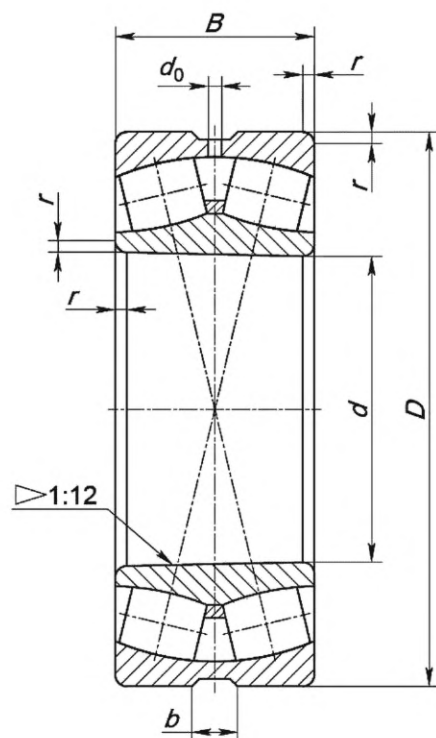
Рисунок 8 — Конструктивное исполнение 15H, серии ширины 0 и 3
